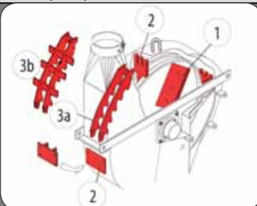
Трехступенчатое измельчение (CH182, CH260 и CH380)
